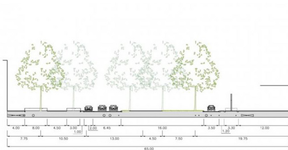
Dwarsdoorsnede van het ontwerp van de Croeselaan. Links is de kant van de woningen, rechts de kantoren.
